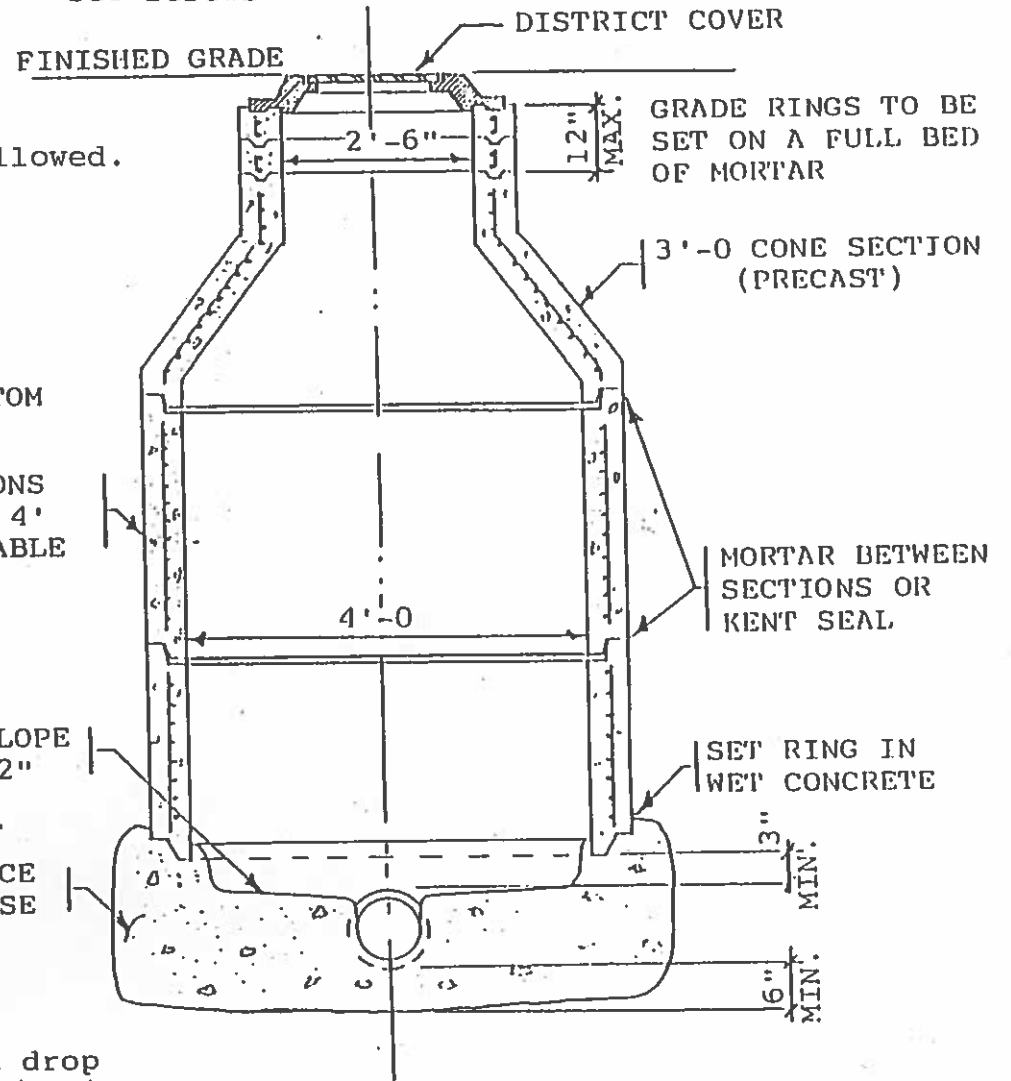
ELEVATION N.T.S.
