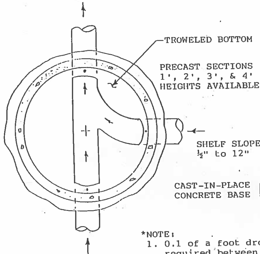
PLAN N.T.S.
